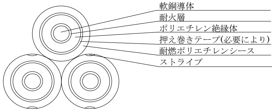
断面図
