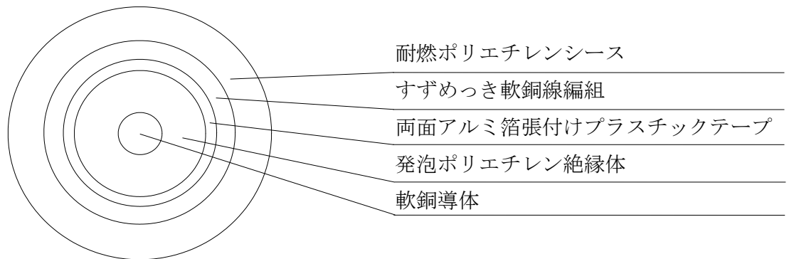
断面図
