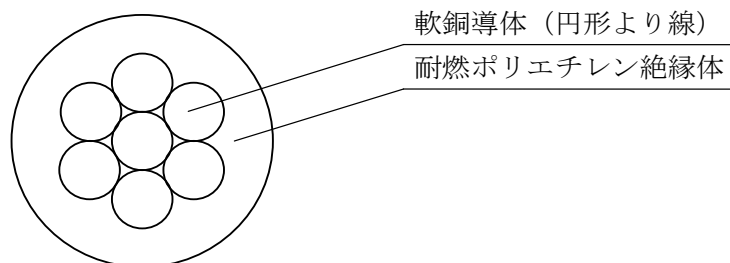
断面図 (より線)
