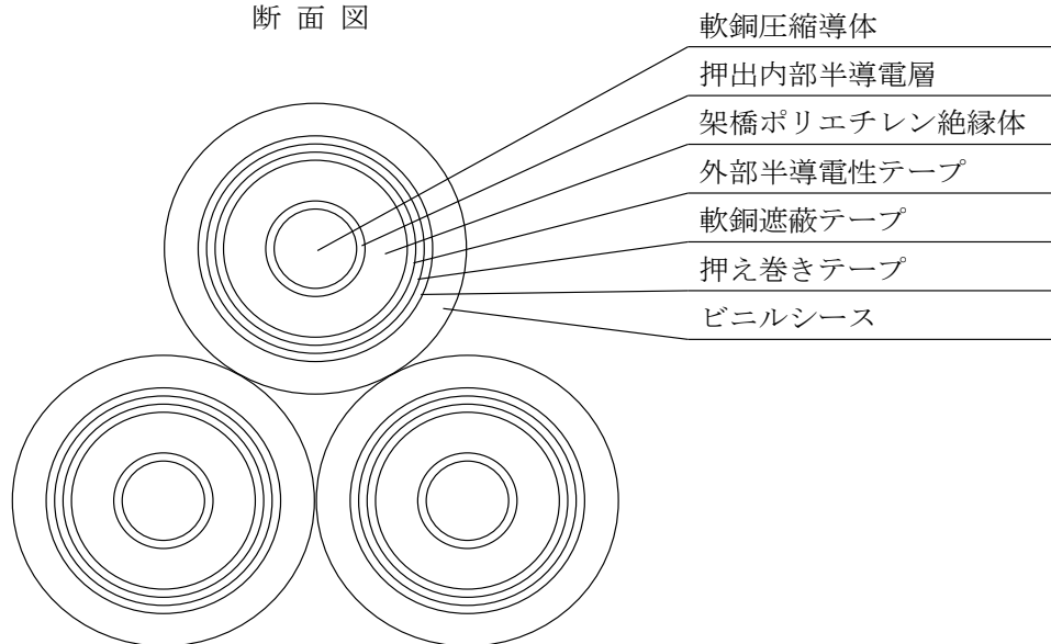
断 面 図
