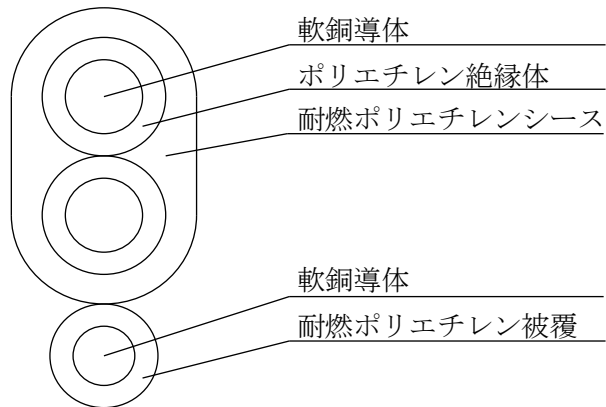
断面図
