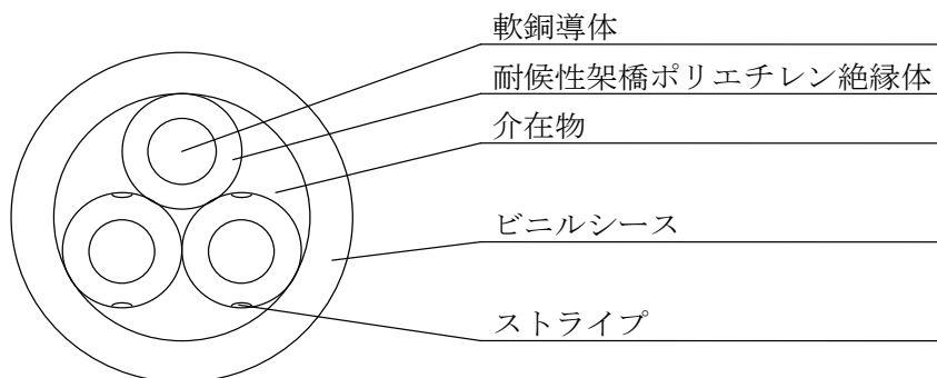
断 面 図
